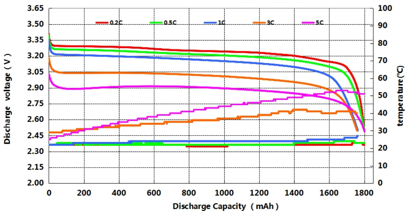
HDCF18650-1800mAh-3.2V (3C) 倍率温升图
