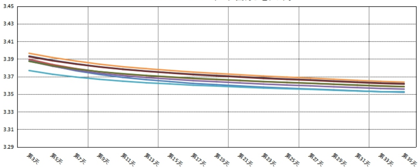
HDCF18650-1800mAh-3.2V(3C) 自放电曲线
