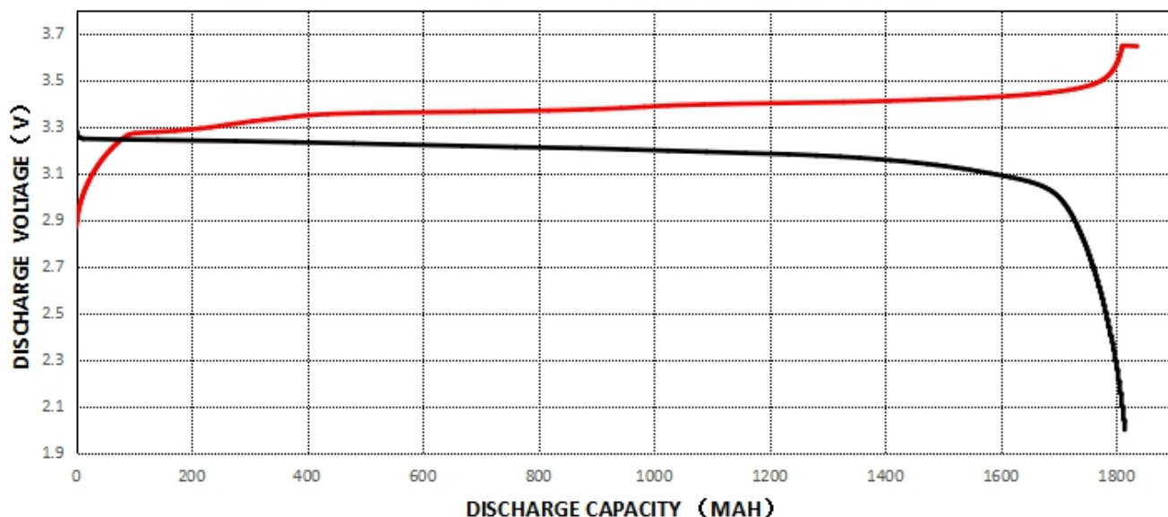
HDCF18650-1800mAh-3.2V(3C) 充放电曲线
