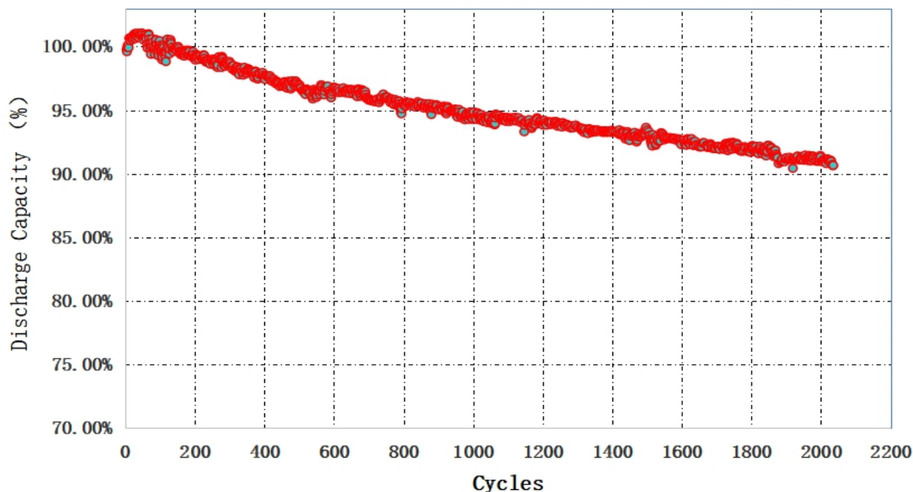
HDCF18650-1800mAh-3.2V (3C) 0.5C/1C循环曲线图
